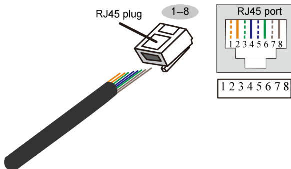
Малюнок 3-24 Обтискна схема дроту Ethernet
