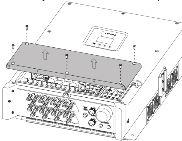
Малюнок 2-23 Демонтаж кришки
