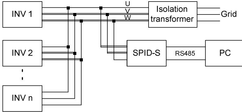
Малюнок 3-30 PLC-з'єднання
