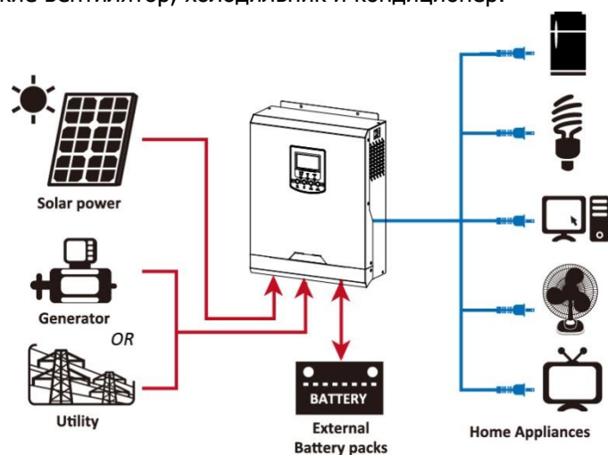
Рисунок 1 Гибридная система электроснабжения
